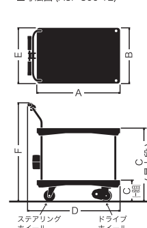
■寸法図 (ASP-300-T2)
