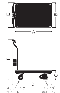
■寸法図 (ASP-300-T2)
