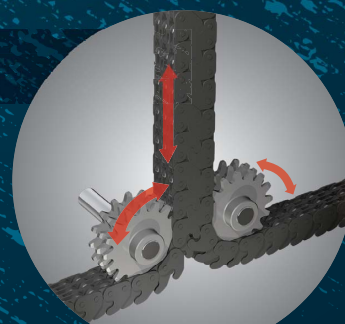
ジップチェーンの構造
